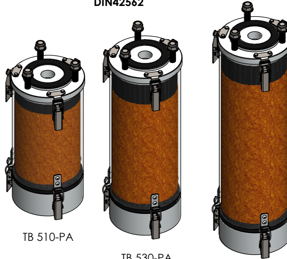
TB 530-PA
